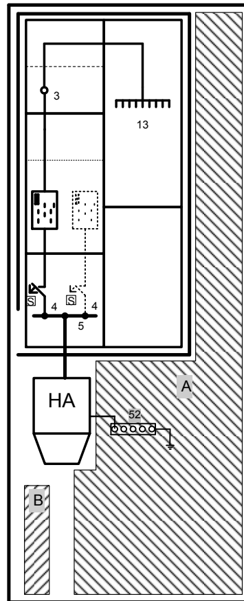
P 2.02 Einkundenanlage (z.B. Einfamilienhaus) für Zählerplatzflächen mit integrierter Befestigungs- und Kontaktiereinrichtung (BKE-I)
